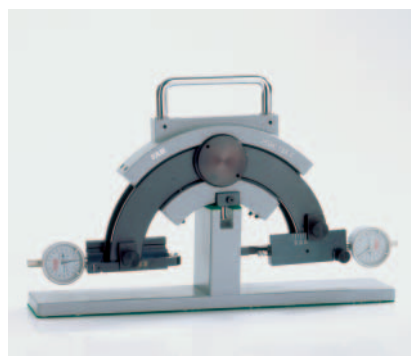
19: Instrumento de medición FAG MGK 133
